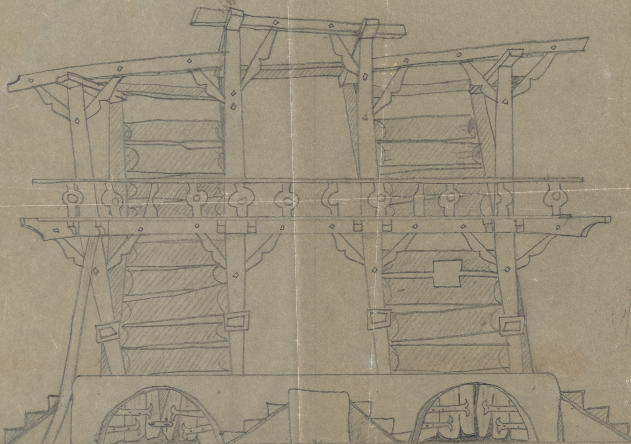
"ŻYWIOT JÓZEFA" WIDOK OGÓLNY 1:25
